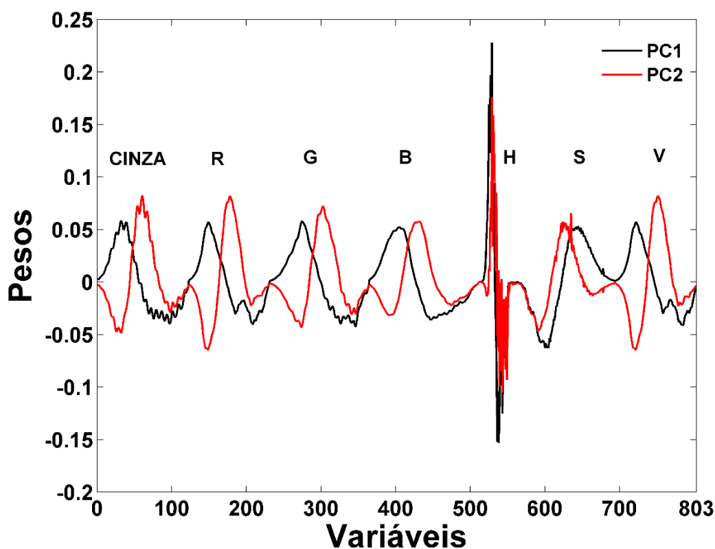
Figura 4.5: Gráfico dos pesos das variáveis em cada componente de cor para o grupo I. R: Red, G: Green, B: Blue, H: Hue, S: Saturação e V: Value.
