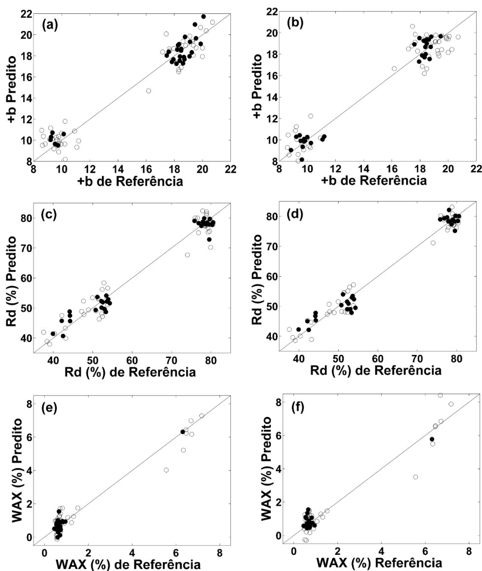
Figura 4.14: Gráfico dos valores preditos versus os valores de referências obtidos pelos modelos PLS (a,c,e) e MLR-SPA (b,d,f) para +b (a-b), Rd (c-d) e WAX (e-f). Amostras de calibração (○) e amostra de predição (●).
