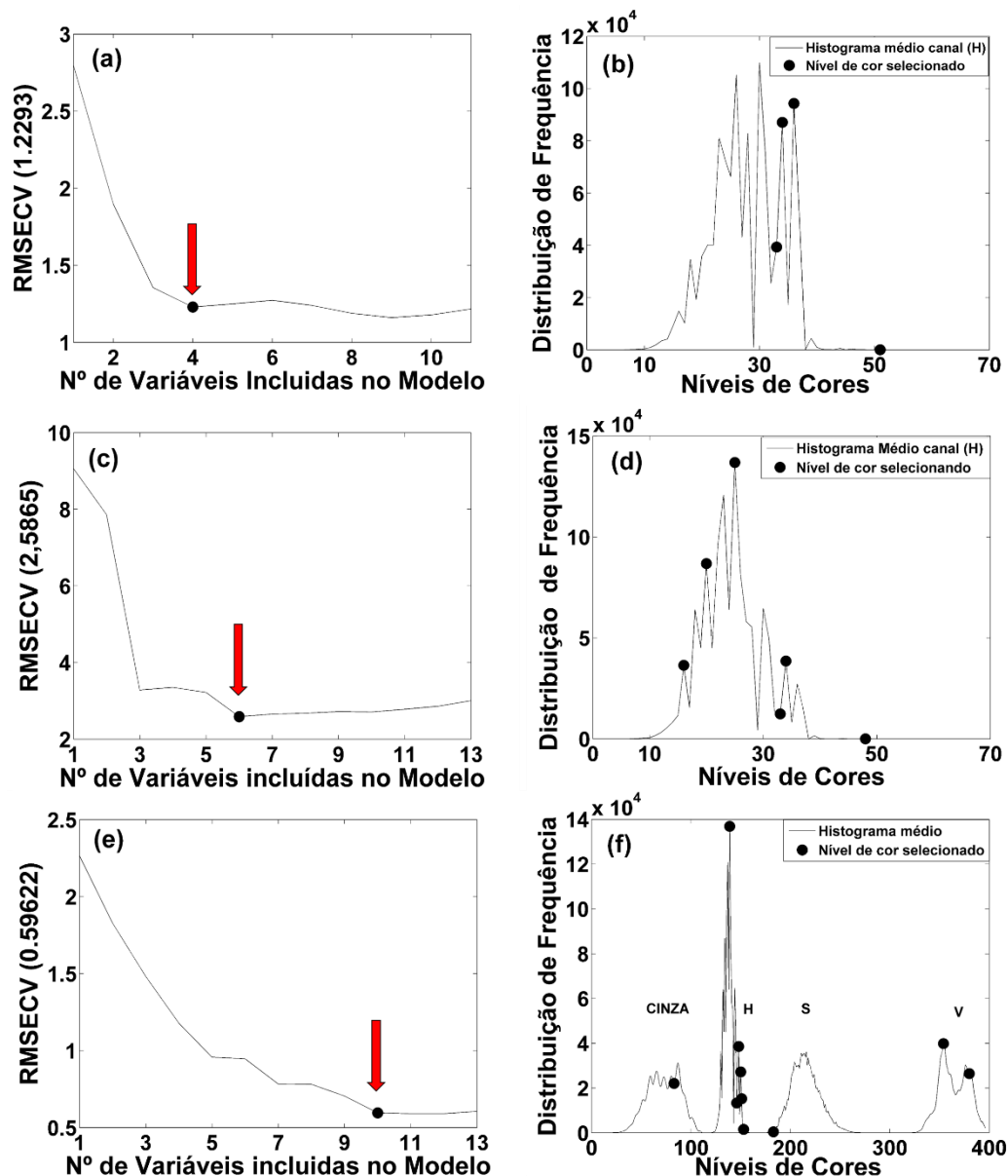
Figura 4.13: Gráficos das variáveis selecionadas versus RMSECV para MLR-SPA (a) +b, (c) Rd e (e) WAX. Histograma médio com as variáveis selecionadas pelo SPA (b) +b, (d) Rd e (f) WAX. As setas identificam o número de variáveis selecionadas.
