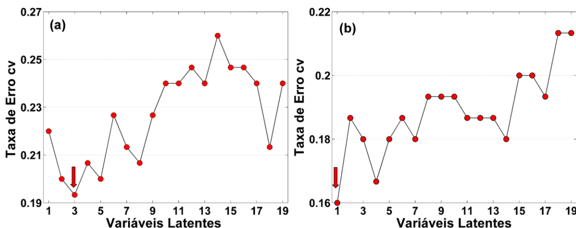
Figura 4.10: Taxa de erro de validação cruzada versus o número de variáveis latentes (a) Grupo I; (b) Grupo II. As setas identificam para o número de variáveis latentes selecionadas.
