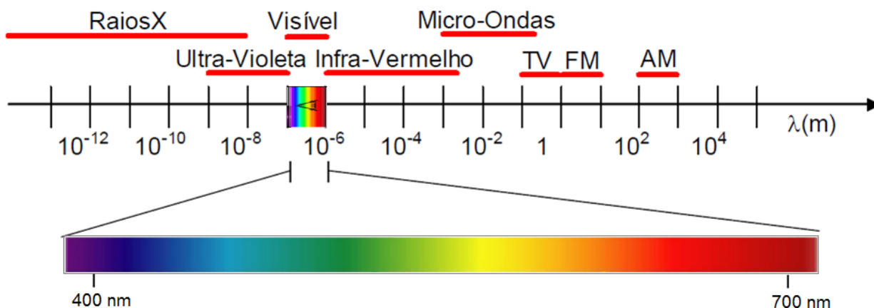
Figura 2.2: Espectro Eletromagnético
