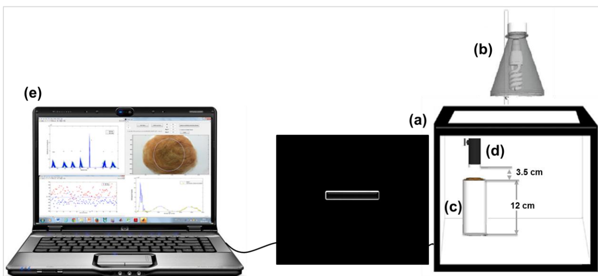
Figura 3.3: Sistema usado na aquisição das imagens de amostras de plumas de algodão naturalmente colorido (a) compartimento, (b) lâmpada fluorescente, (c) suporte de Teflon ®, (d) webcam e (e) notebook
