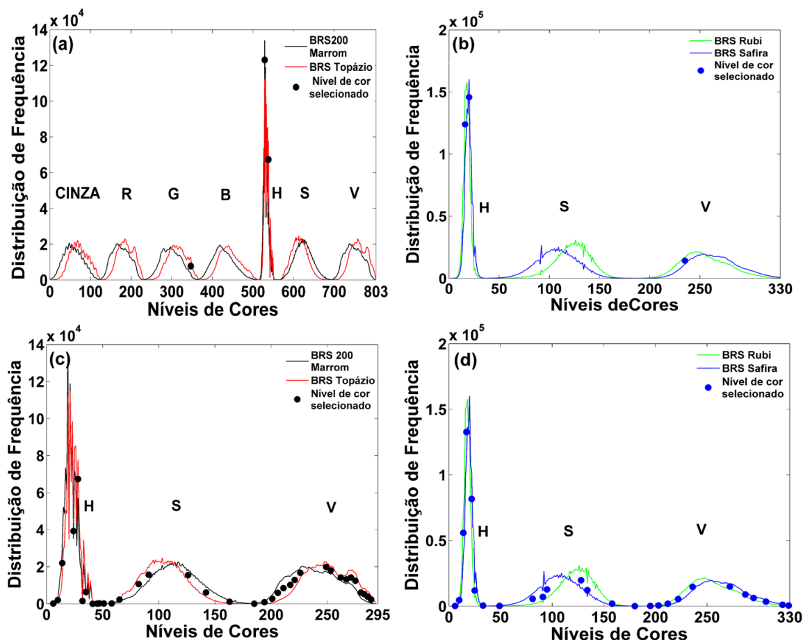
Figura 4.8: Média dos histogramas para cada cultivar, com as Variáveis selecionadas (●, ●) pelo LDA/SPA (a e b) e pelo LDA/SW (c e d) para o Grupo I (a e c) e Grupo II (b e d).
