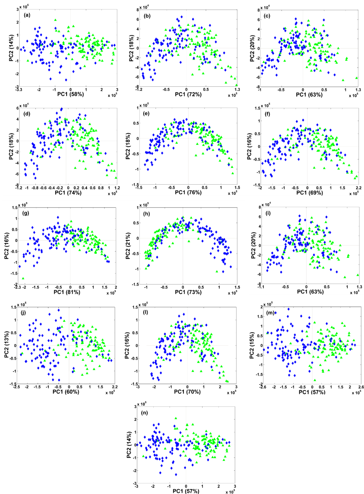
Figura 4.6: Gráfico dos escores obtidos pela PCA aplicada aos histogramas do grupo II ( \blacktriangle : BRS Rubi, \blacklozenge : BRS Safira). (a) todos os canais; b) tons de cinza; c) R, (d) G, (e) B, (f) RGB, (g) H, (h) S, (i) V, (j) HSV, (l) Cinza-RGB, (m) Cinza-HSV, (n) RGB-HSV. A variância explicada para cada PC é encontrada entre parêntese.
