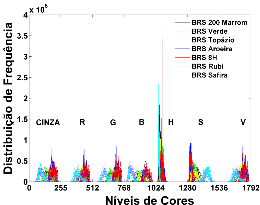
Figura. 4.11: Histogramas completos, das plumas de algodão. R: Red, G: Green, B: Blue, H: Hue, S: Saturation e V: Valor.
