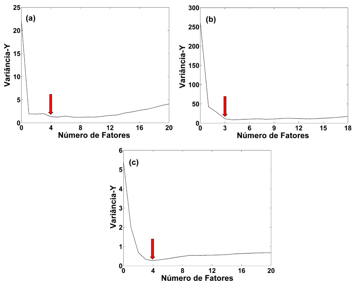
Figura 4.12: Gráfico da variância em y versus o número de fatores dos modelos PLS, para (a) +b, (b) Rd e (c) WAX.
