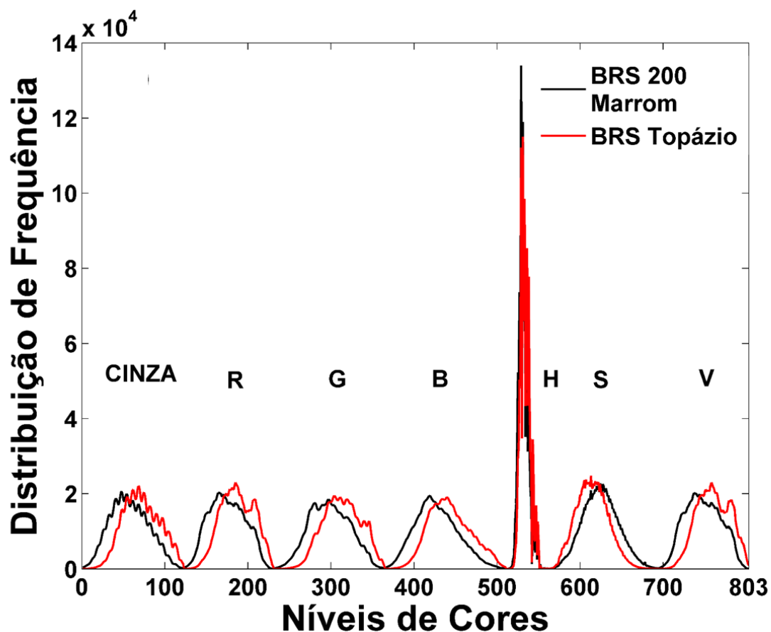
Figura 4.2: Histograma médio para o grupo I. R: Red, G: Green, B: Blue, H: Hue, S: Saturation e V: Value.
