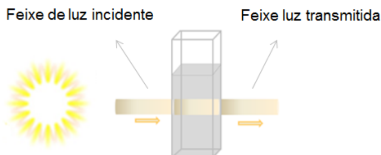
Figura 2.4: Transmissão da luz
